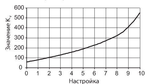
Расходная характеристика
